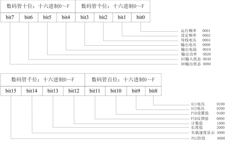
图 5-17. LED 运行显示位对应图
