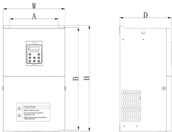
图 2-6. (4T) 45~132KW 变频器外型尺寸及安装尺寸示意图 (7T) 30~55KW 变频器外型尺寸及安装尺寸示意图
