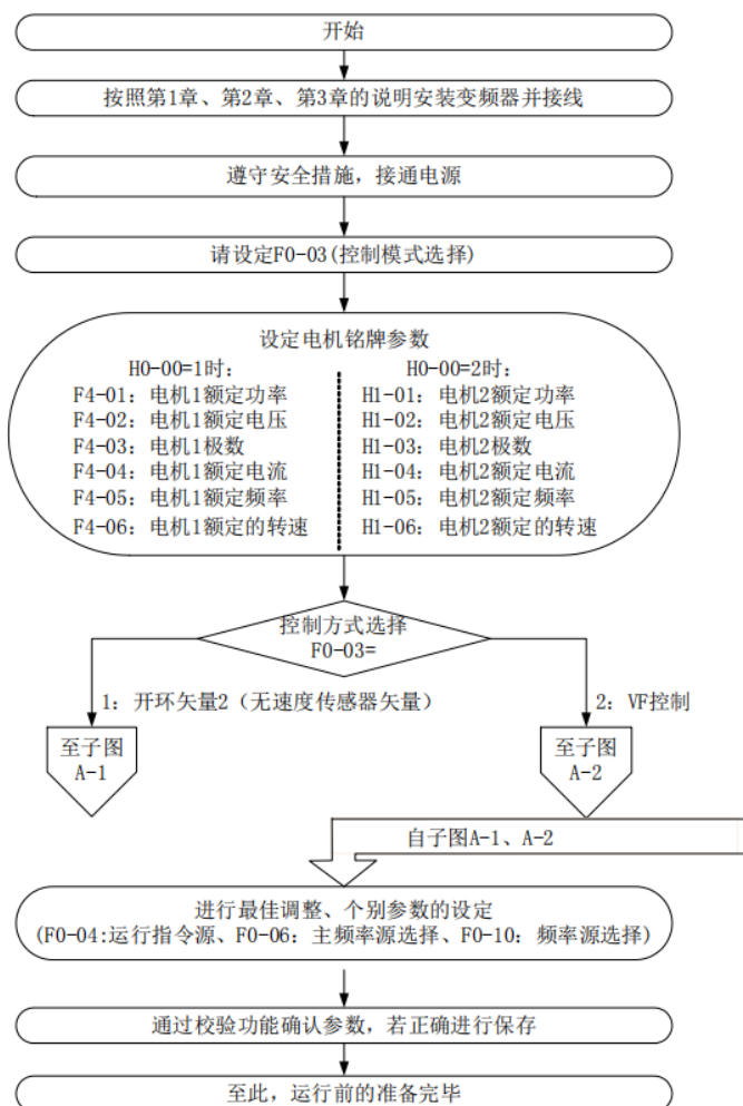
图 4-5. 运行前的基本步骤
