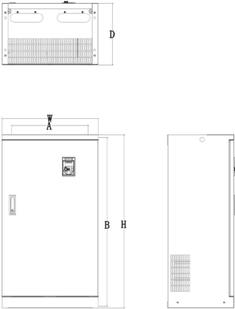
图 2-7. (7T) 75KW 以上变频器外型尺寸及安装尺寸示意图
