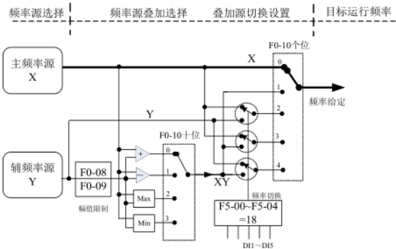
图5-1. 频率源叠加示意图
