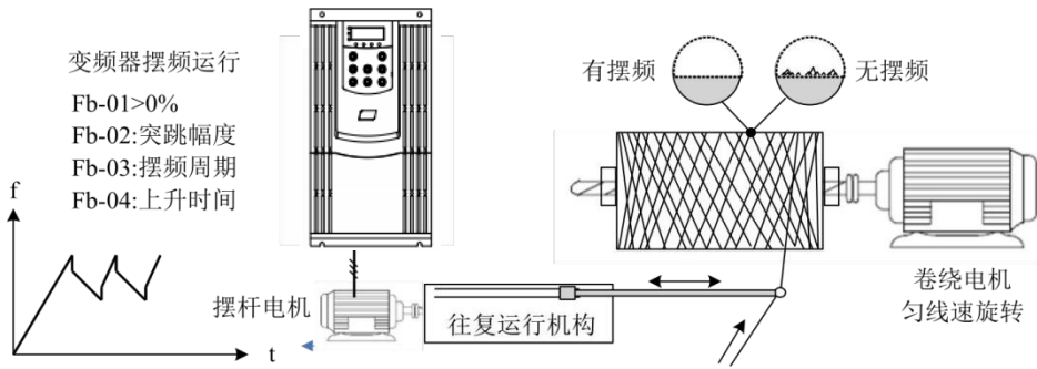
图4-20. 摆平运用设置示意图
