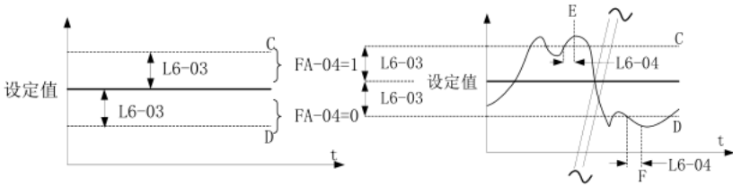
图5-33. 唤醒示意图
