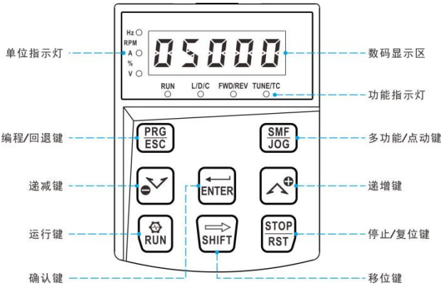
图4-1. 操作面板示意图1(标准配置LED键盘)
