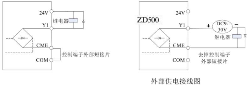
图3-13.数字输出端子Y1接线示意图
