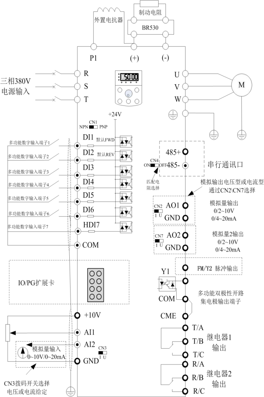
图 3-9. (4T)75Kw 及以上三相变频器
