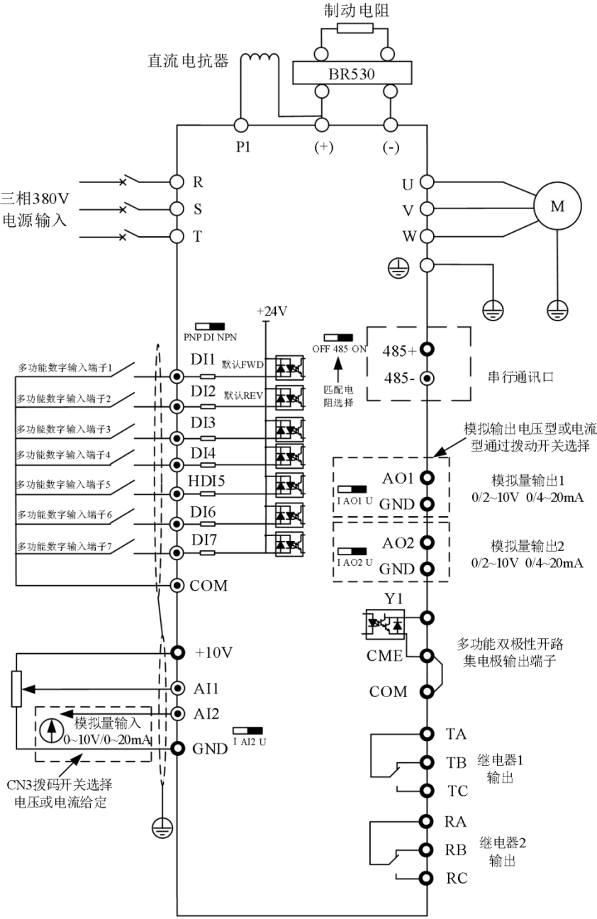
图 3-10. (7T) 75Kw 及以上三相变频器
