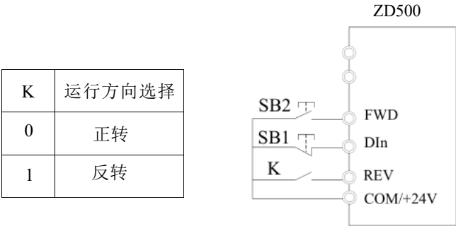
图 5-10. 三线式运转模式 2
