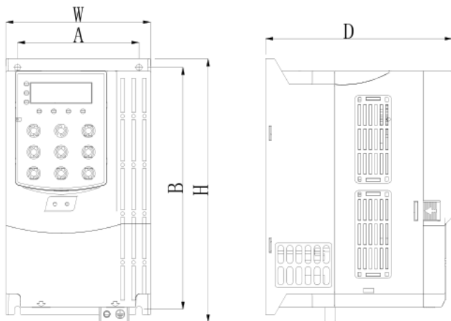
图 2-3.(3S/4T) 7.5KW 以下塑胶外形尺寸及安装尺寸示意图
