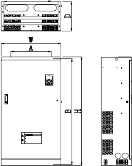
图 2-7. (4T) 160KW 以上变频器外型尺寸及安装尺寸示意图
