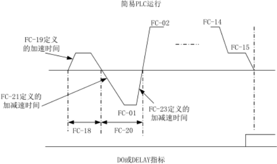
图5-29. 简易PLC示意图
