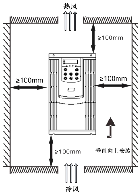
图3-1. 单体安装图
