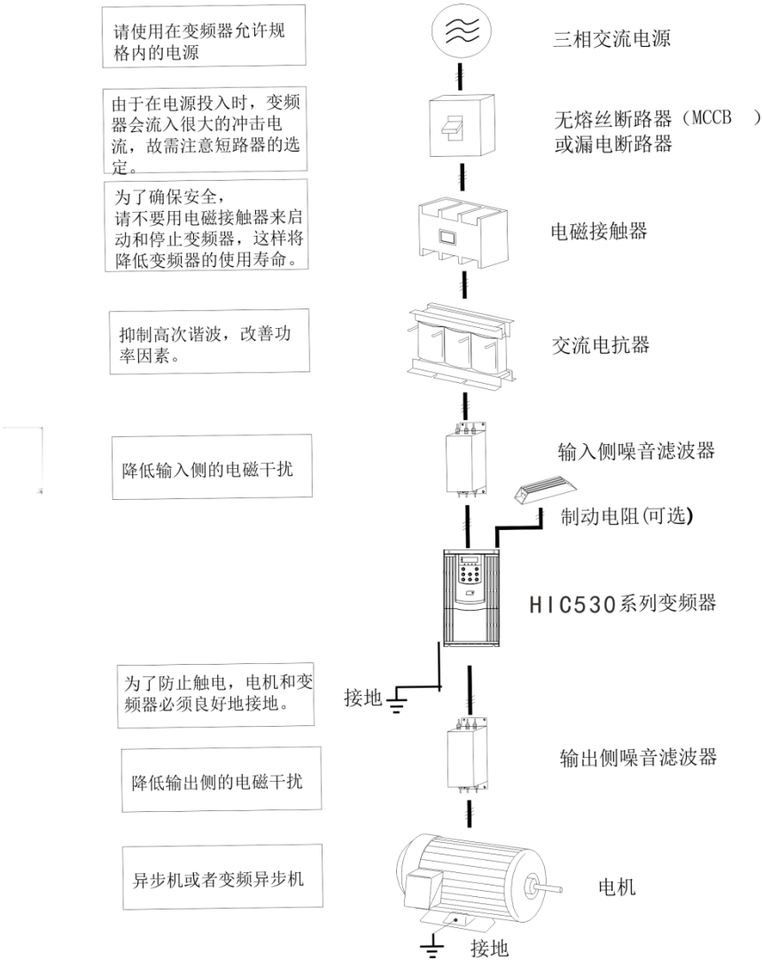
图 1 与外围机器的连接示例
