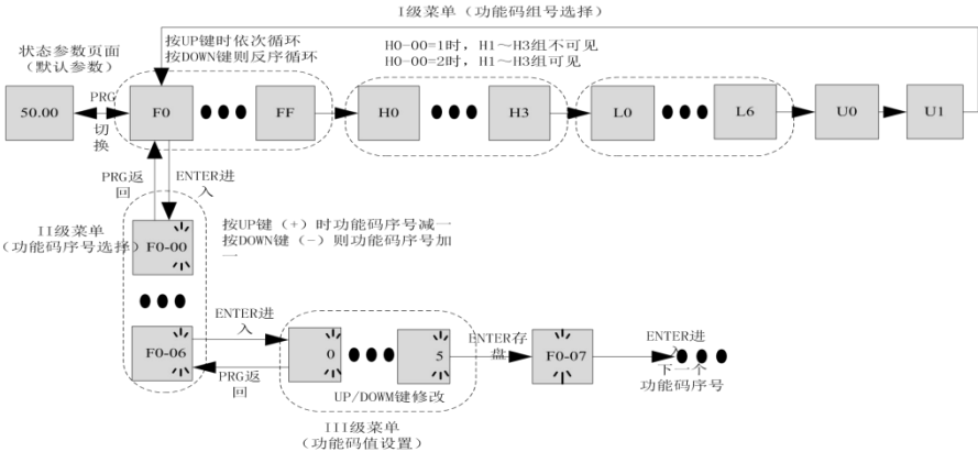
图4-2. 三级菜单操作流程图
