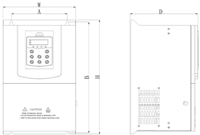
图 2-5. (4T) 18~37KW 钣金机箱外形尺寸及安装尺寸示意图 (7T) 11~15KW 钣金机箱外形尺寸及安装尺寸示意图
