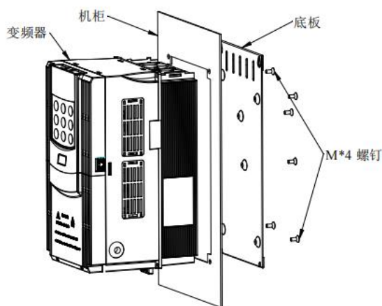
图3-3. ZD500变频器塑胶结构穿墙式安装图
