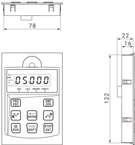
图 2-6.外引键盘带托盘安装尺寸图
