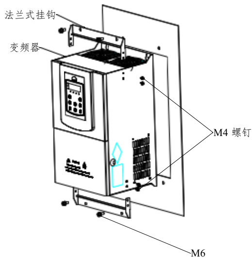
图3-4. ZD500变频器钣金结构穿墙式安装图
