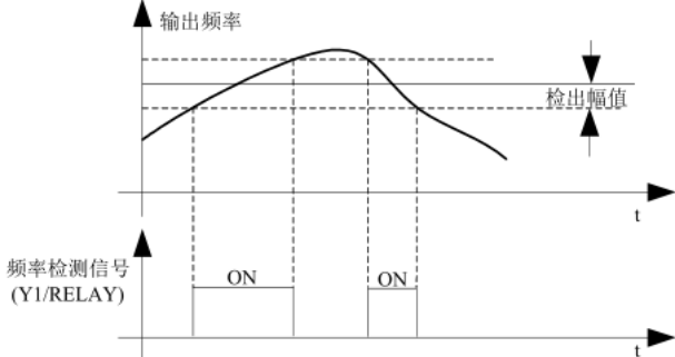
图 5-16. 频率到达检出幅值示意图
