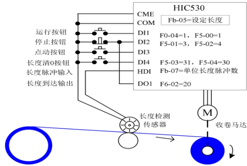
图 4-24. 定长控制功能常见应用举例
