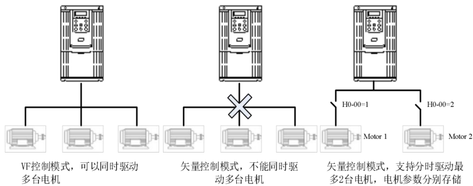
图 4-26. 多组电机的切换
