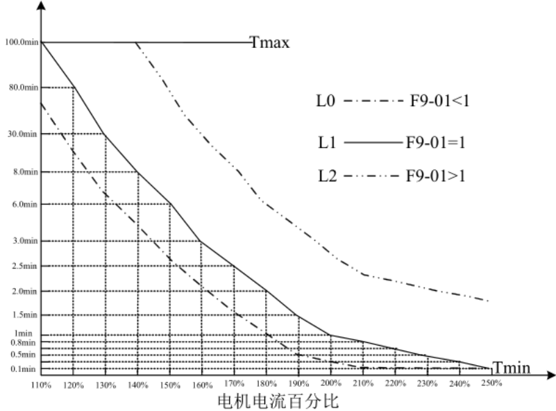
图5-21. 电机过载保护曲线
