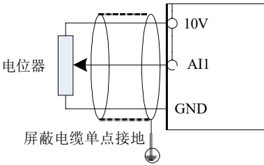
图 3-11.模拟量输入端子接线示意图
