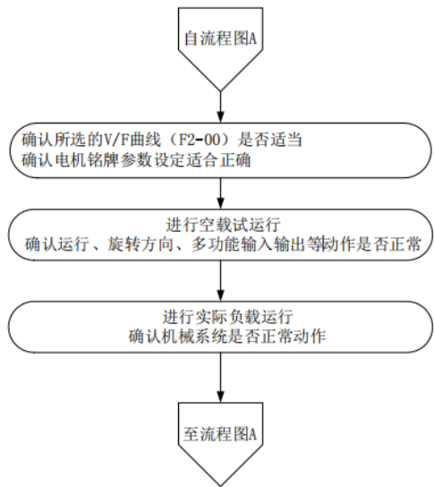
图 4-7. V/F 控制方式运行步骤
