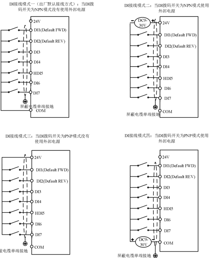
图3-12. 四种不同模式下数字输入端子接线图
