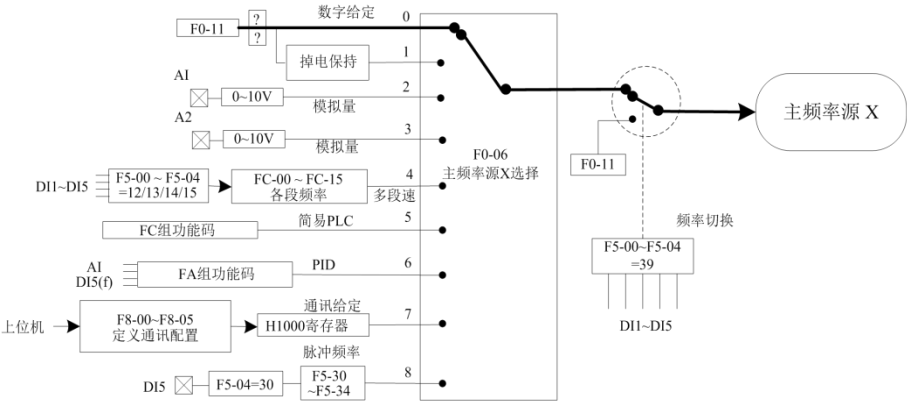
图4-17. 主频率源X设置示意图
