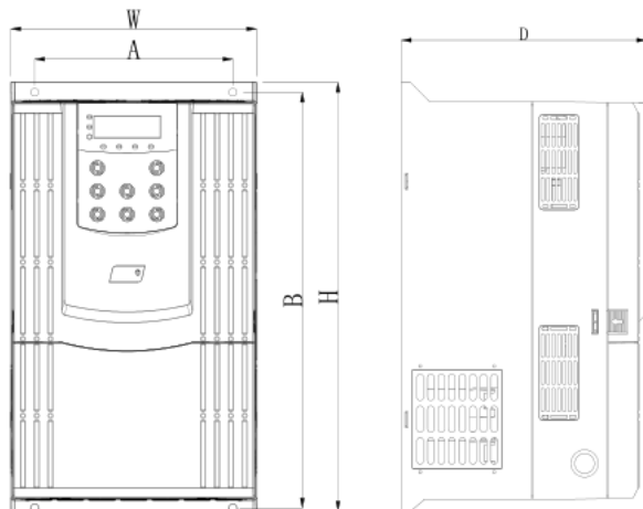
图 2-4. (4T)11~15KW 塑壳机箱外形尺寸及安装尺寸示意图
