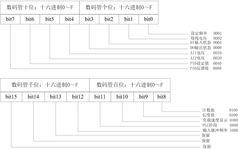
图 5-18. LED 停机显示对应图
