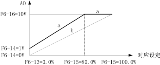
图4-29. A0输出示意图
