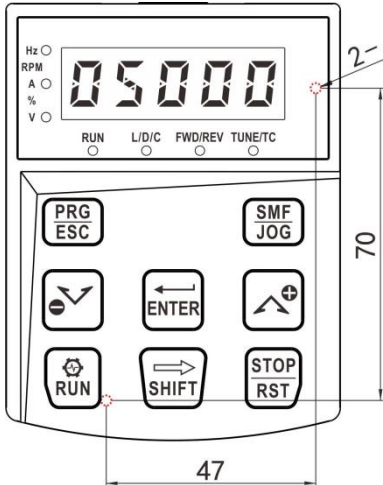
图 2-5.外引键盘不带托盘安装尺寸图
