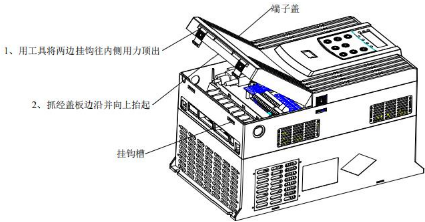
图3-5. 塑胶外壳端子盖拆卸图
